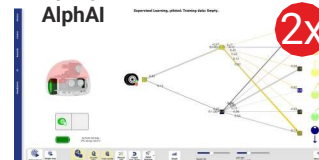
Oprogramowanie AlphAI
